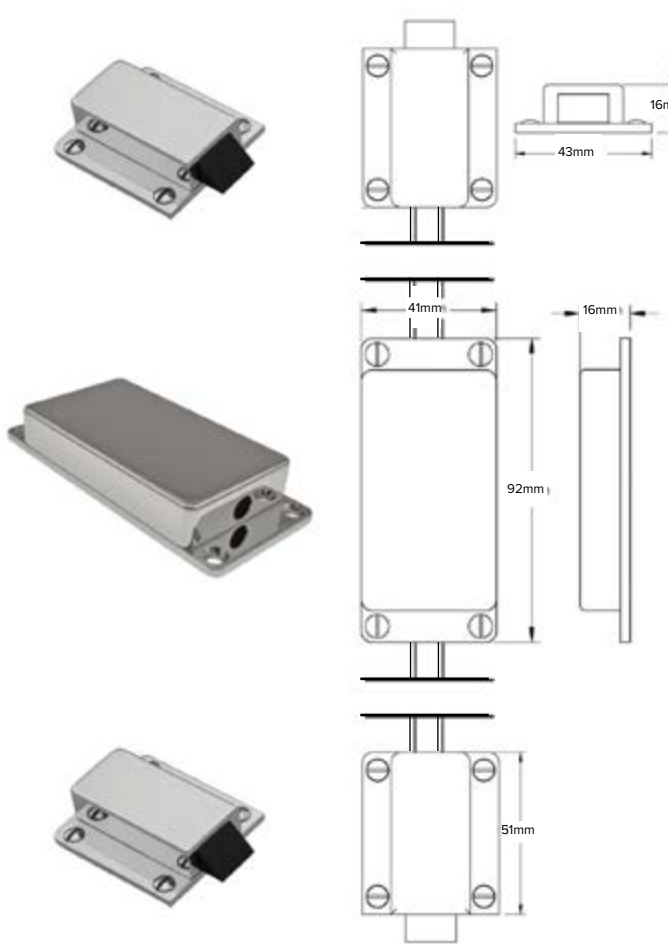
Turning Lux Slam Espagnolette PLK232
