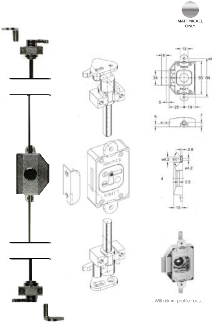
Standard Turning Espagnolette PLK360
