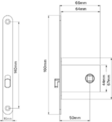
Sliding door privacy lock K1500
